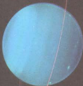
Уран
